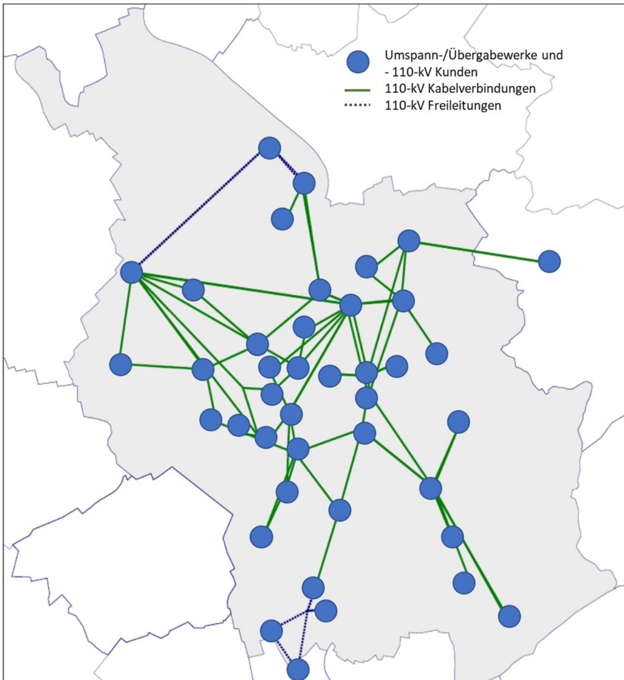
Anlage 1: Stromnetzkarte
